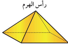
هرم رباعي القاعدة
