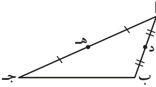
مثلث منفرج الزاوية
