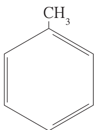
ميثيل البنزين (الطولوين)
