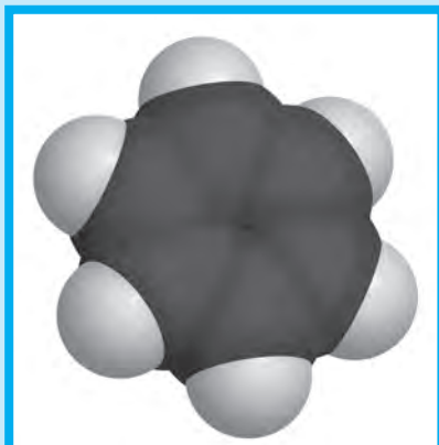
شكل (35) نموذج التعبئة المجسّمة للبنزين
