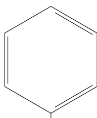
CH_3 - CH_2 - CH - CH_2 - CH_2 - CH_3 3- فينيل الهكسان
