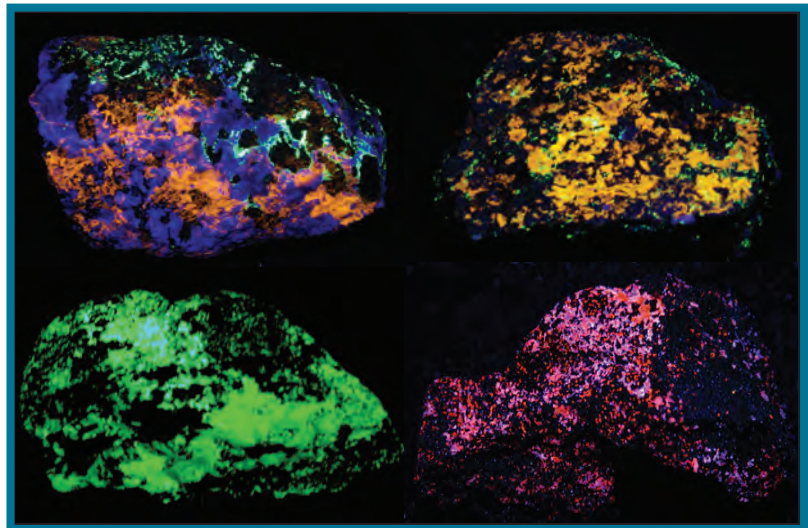
شكل 39 بعض المعادن المتضيؤة
