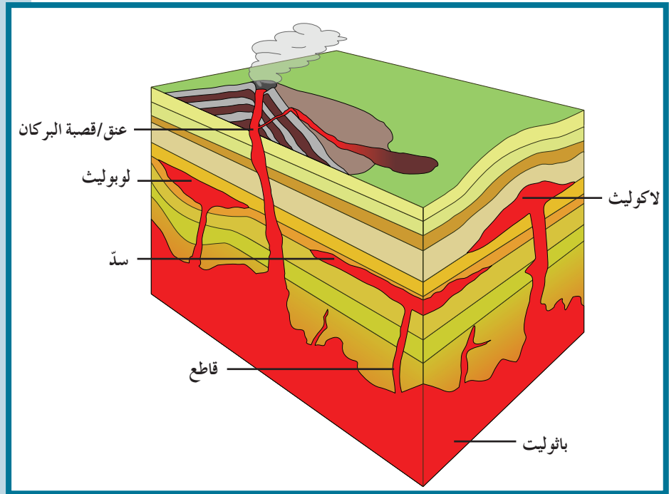
شكل 64 أشكال صخور النارية في الطبيعة.
