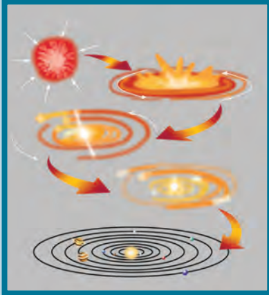
شكل 15 مراحل المجموعة الشمسية
