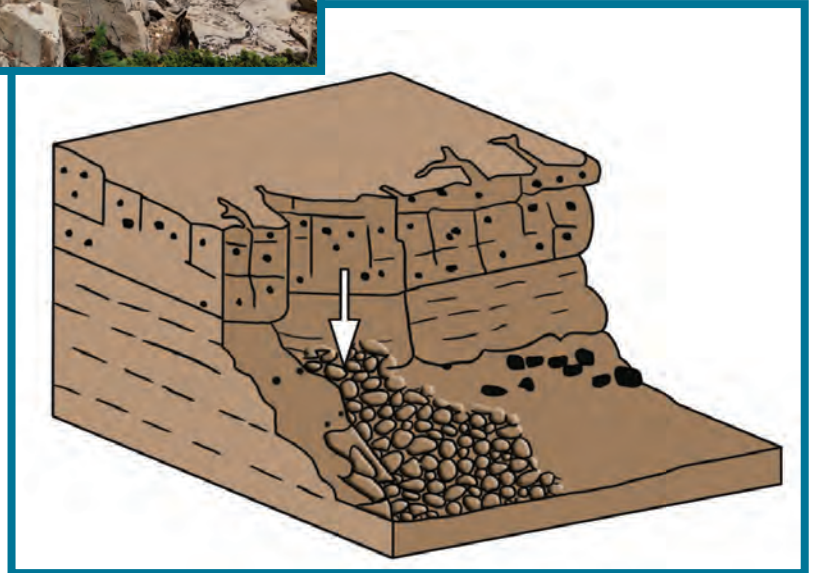
شكل 128 التساقط من المنحدرات الشديدة
