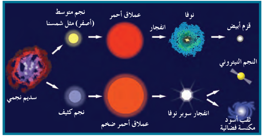
شكل 11 دورة حياة النجوم
