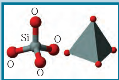
شكل 47 التركيب البنائي لجميع المعادن السيليكاتية
