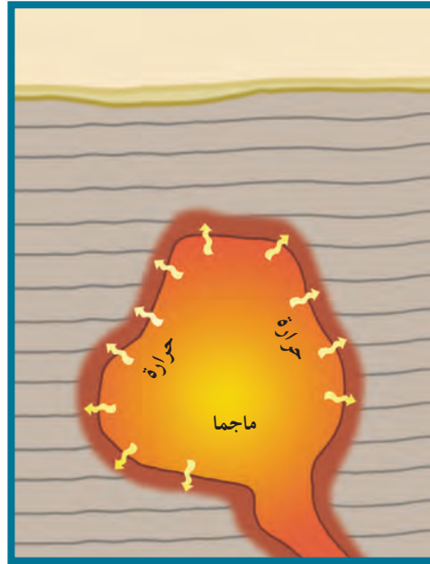
شكل 115 هالة التحوّل
