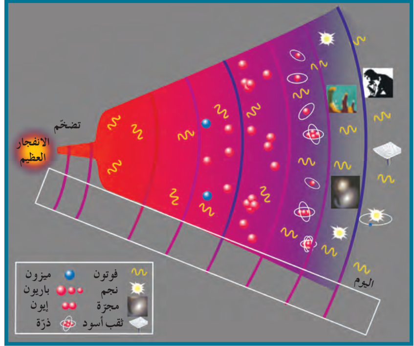
شكل 5 نشأة الكون
