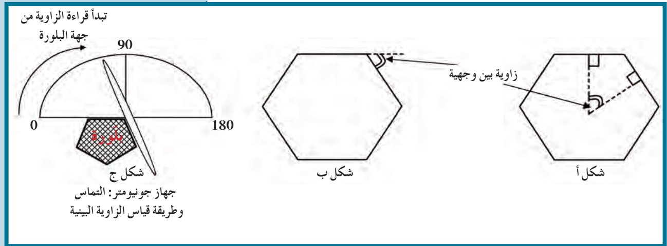
شكل 52 زاوية بين وجهية
