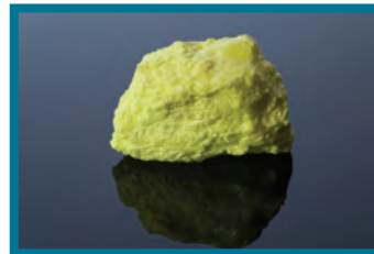
شكل 22 معدن الكبريت
