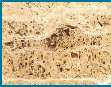
شكل 79 الترافرتين
