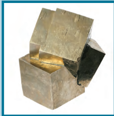
شكل 54 بلورات توأمية
