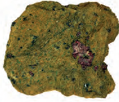
شكل 67 صخرة البريدوتيت
