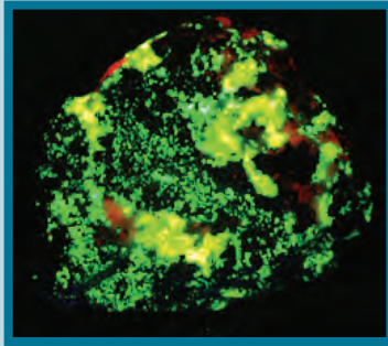
شكل 40 معدن الويليميت
