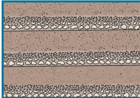
شكل 94 التطبق المتدرج
