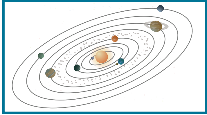
شكل 14 المجموعة الشمسية
